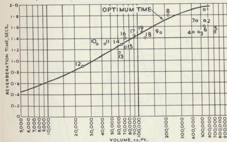
Abb. 2 Verhältnis von optimaler Nachhallzeit und Volumen (Nachhallzeiten bei Anwesenheiten von Orchester und — soweit anwendbar — Publikum)
