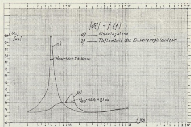
Abb. 3 Scheinwiderstandsverlauf a) bei einem Lautsprechersystem b) bei vier Systemen. Fig. 3 Impedance characteristic a) for one loudspeaker b) for four loudspeakers
