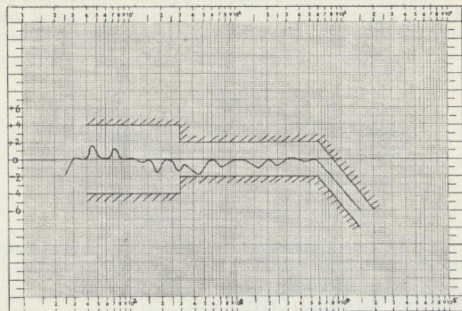
Abb. 2 Genormte Schalldruckkurve des Einheitsregielausprechers. Fig. 2 Standard response curve of the new loudspeaker for control booths.
