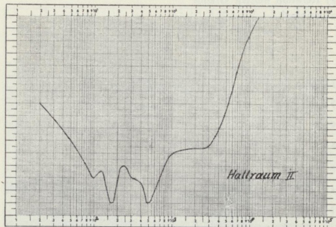
Abb. 5 Betriebsmäßiger Verlauf von zwei Entzerercurven für verschiedene Räume.
