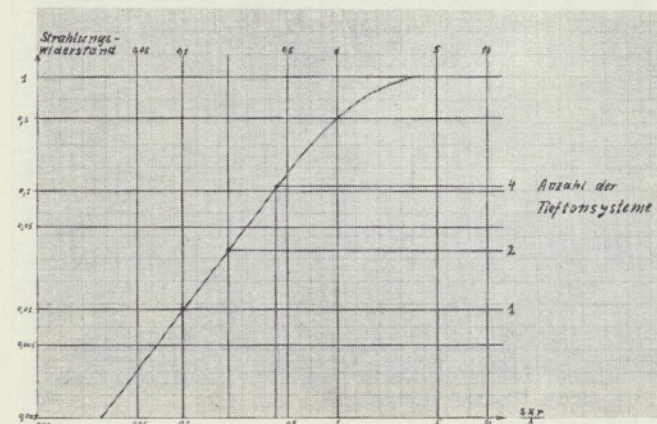
Abb. 1 Abhängigkeit des Strahlungswiderstandes von der Größe der schwingenden Fläche.
