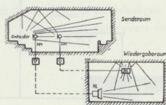
Fig. 22 Zwei Kanal-Übertragung mit einem besonderen Raummikrofon nach Buttenberg
