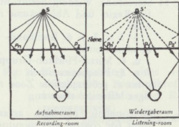
Fig. 10 Raumbezügliche Übertragung mit zwei Hilfsebenen (nach Fletcher) Fletcher's stereophony with one imaginary plane 1 in the recording-room at the left, and another 2 in the listen- ing-room at the right
