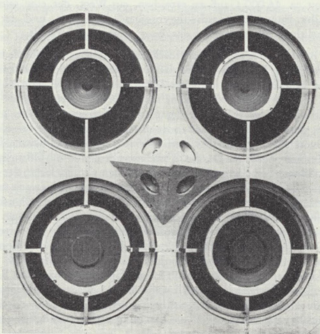
Abb. 1 Lautsprecher-Kombination für höchste Wiedergabetreue, bestehend aus vier Tieftön-, vier Mittelton- und vier Hochton-Lautsprechern.
