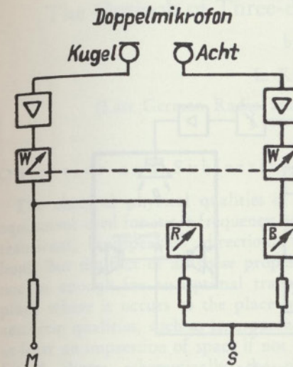
Fig. 17 Prinzipschaltung eines vollständigen Stereomikrofonkanals mit Basis und Richtungsregelung W = gekoppelte Mikrofonmischregler
