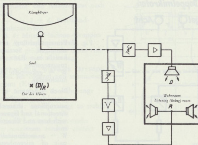
Fig. 20 Schema für die Abbildung des D/R -Verhältnisses des Ursprungsraumes in den Wiedergaberaum
