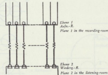
Fig. 11 Vereinfachte raumbezügliche Übertragung mit n Kanälen (nach Warncke) Simplified stereophony with two imaginary planes 1 and 2 and a finite number of n channels (Warncke)
