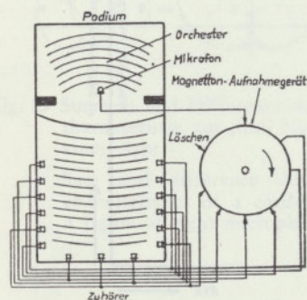
Fig. 21 Stereonachhallanlage von Philips Philips's Ambiphony
