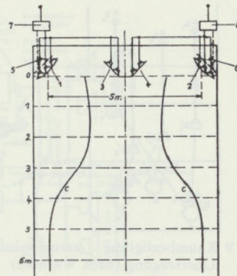
Fig. 14 Stereofone Wiedergabeeinrichtung für Regie- und Abhörräume nach Kuhl
