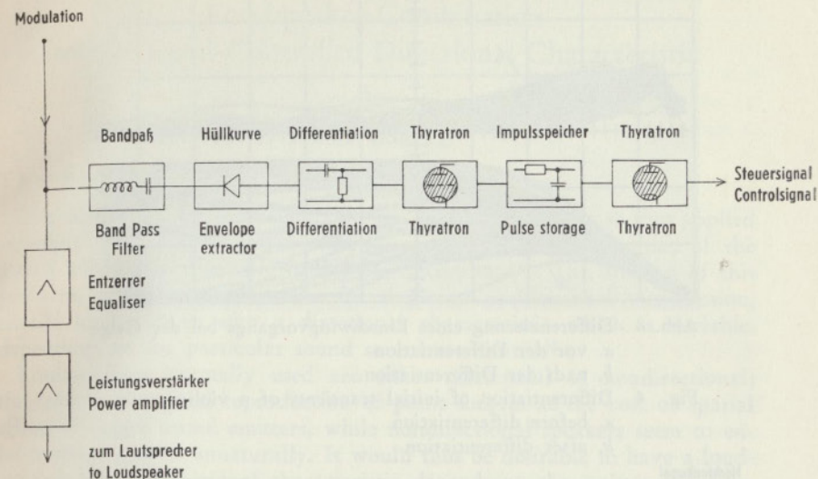
Abb. 2 Blockschaltbild der Einrichtung zur elektronischen Differentiation von Schallkurven.
