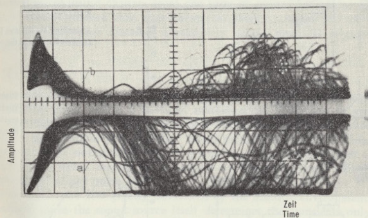
Abb. 3 Differenzierung eines Einschwingvorgangs bei Sprache a. vor der Differentiation b. nach der Differentiation.
