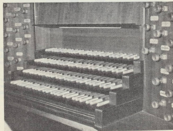
Abb. 2 Manuale und Registerzüge im Spielschrank der Orgel. Von unten nach oben: Rückpositiv, Hauptwerk, Oberwerk und Schwellwerk.
