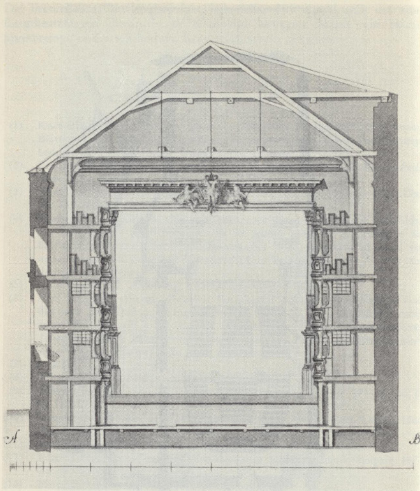
Querschnittsdarstellung von der Linie A — B des Grundrisses gegen die Bühne, 1779. (Albertina, Architektur Inv.-Nr. 6573).
