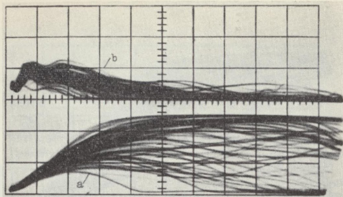
Abb. 4 Differenzierung eines Einschwingvorgangs bei der Geige a. vor der Differentiation b. nach der Differentiation.
